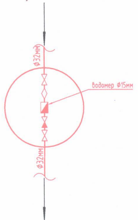
Схема водомерного узла BK-2
